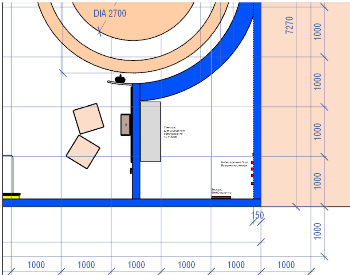
Схема подсобного помещения (серверная)
